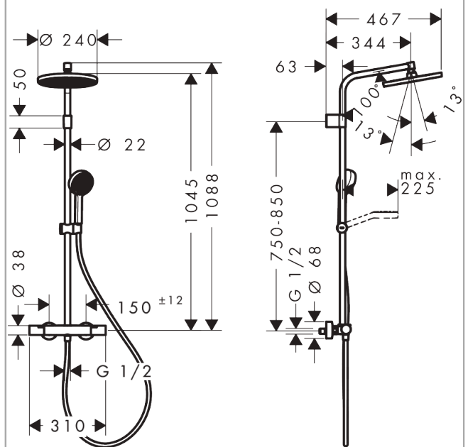
Maattekening
