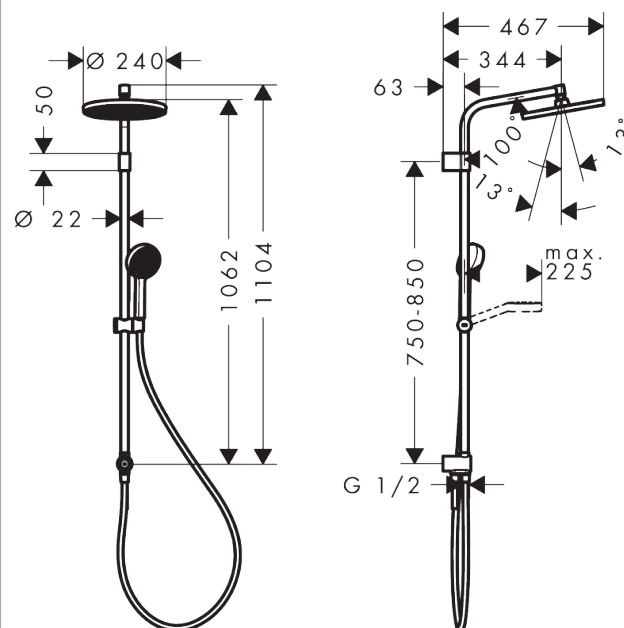
Maattekening
