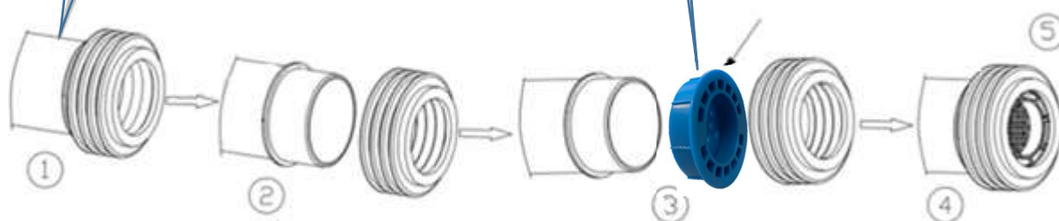
honingraatbegrenzer
