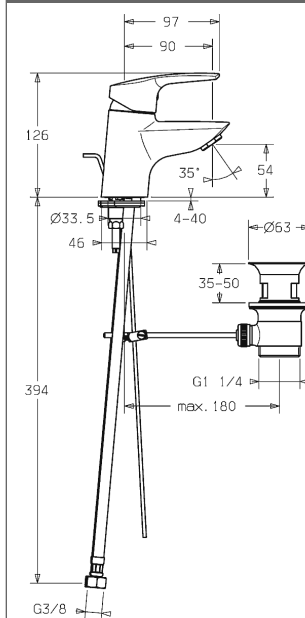
Producttekening
